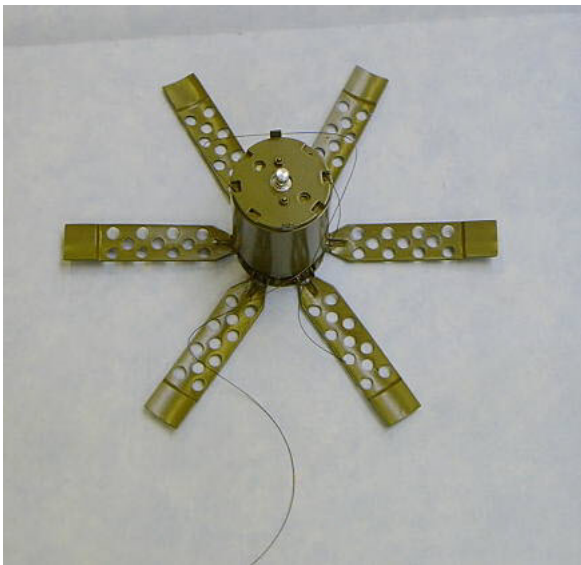
POM-2S p/number: TSUB-012
